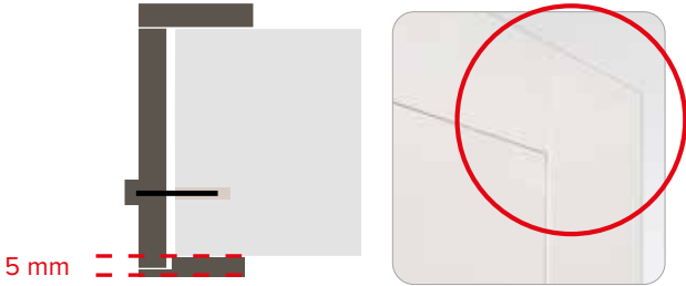
Deurgeheel met gelijkliggende deurlijsten. Bloc-porte avec chambranles au même niveau que la porte.
