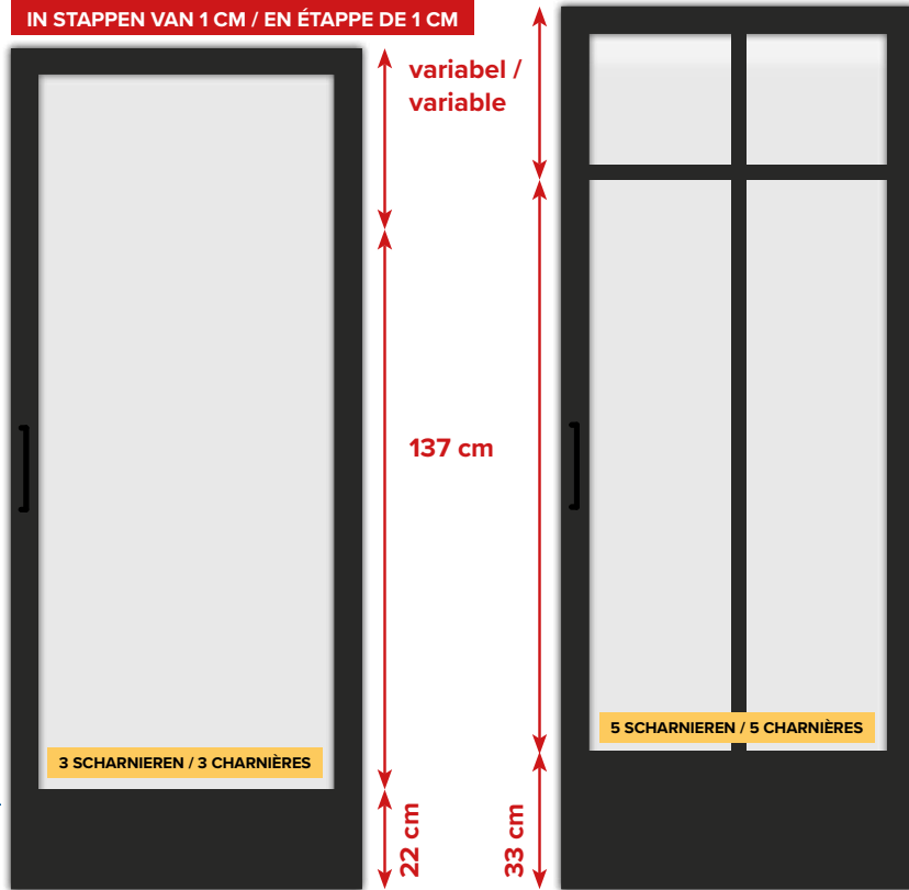
Steel Feeling - PAN1R 180 cm - 201 cm - op maat / sur mesure
